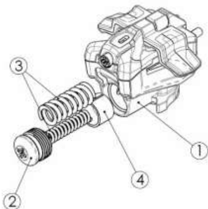
Obrázek 1 – demontáž kalibrované patky
