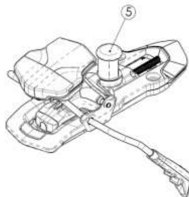
Obrázek 2 – patní základová deska (baseplate) s brzdou
